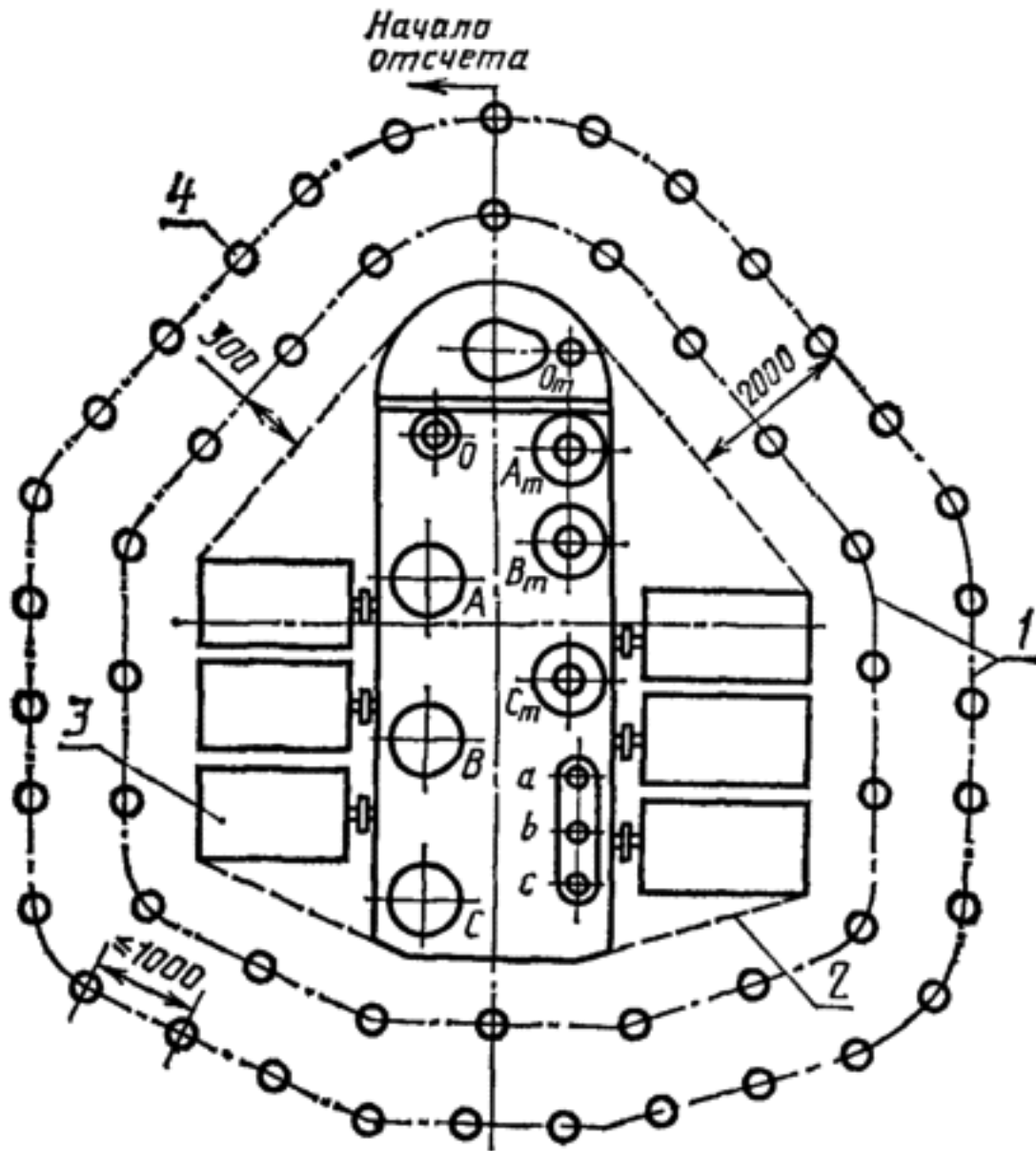
1 — измерительная линия; 2 — излучающая поверхность; 3 — охладители; 4 — микрофон
