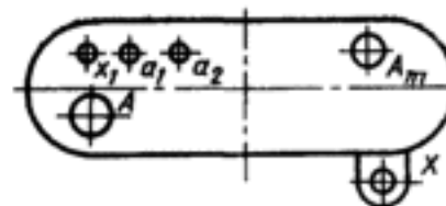
б) автотрансформатор АОДЦТН-417000/750/500
