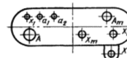
а) автотрансформатор АОДЦТН-333000/750/330
