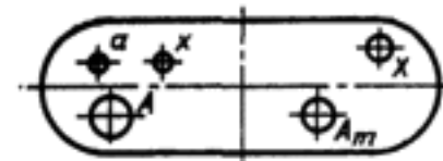
а) автотрансформатор АОДЦТН-267000/750/220
