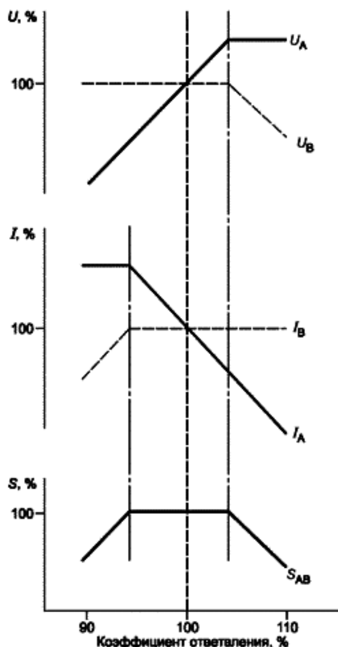
Рисунок 3 — Комбинированное регулирование напряжения (режим a )
