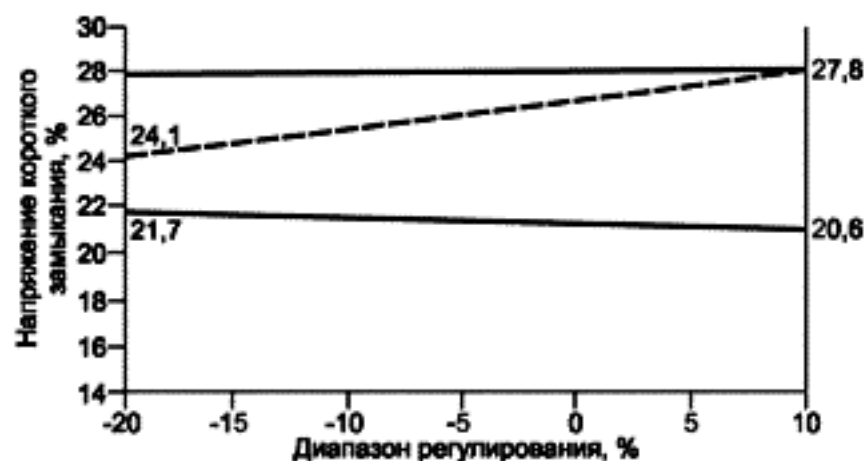
Рисунок В.1 — Диапазон изменения напряжения короткого замыкания
