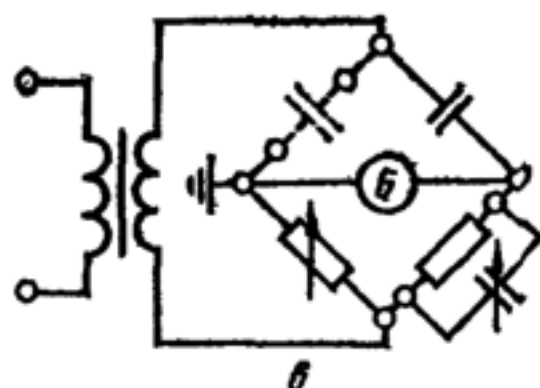
Схема с заземленной диагональю
