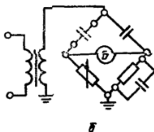
Схема с заземленной диагональю
