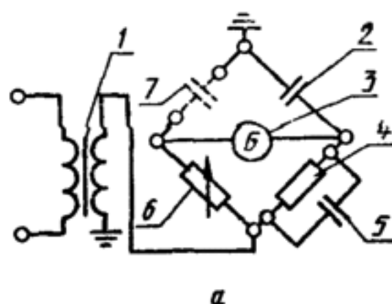
Схема с заземленной диагональю
